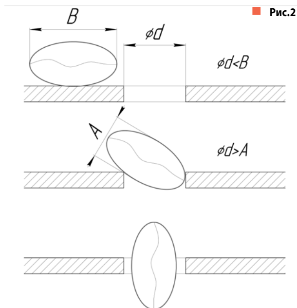
Рис. 2. Схема прохода частицы в круглое отверстие.
