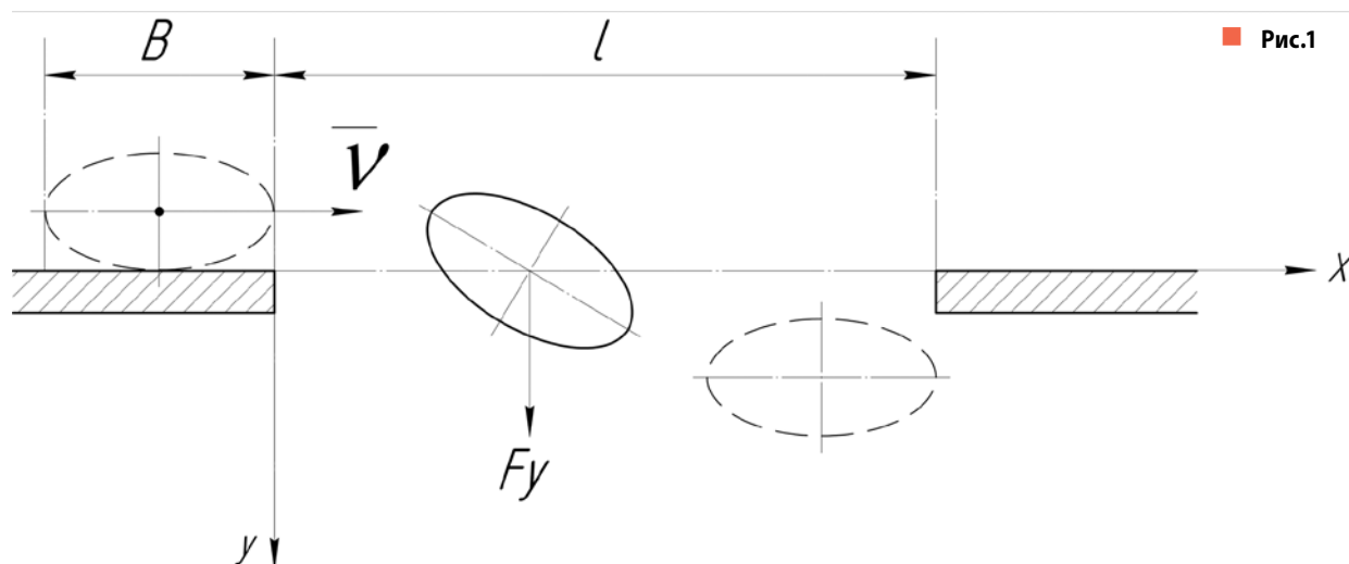
Рис. 1. Схема к определению условий выделения проходовой частицы.
